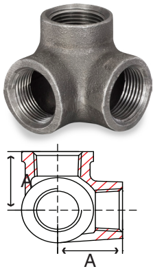
Fig. 330E1 & 340E1 – 90° Side Outlet Elbow
