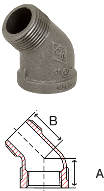
Fig. 33SF1 & 34SF1 – 45° Street Elbow
