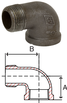
Fig. 33SE1 & 34SE1 – 90° Street Elbow
