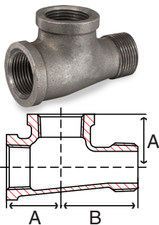
Fig. 33ST1 & 34ST1 – Service Tee
